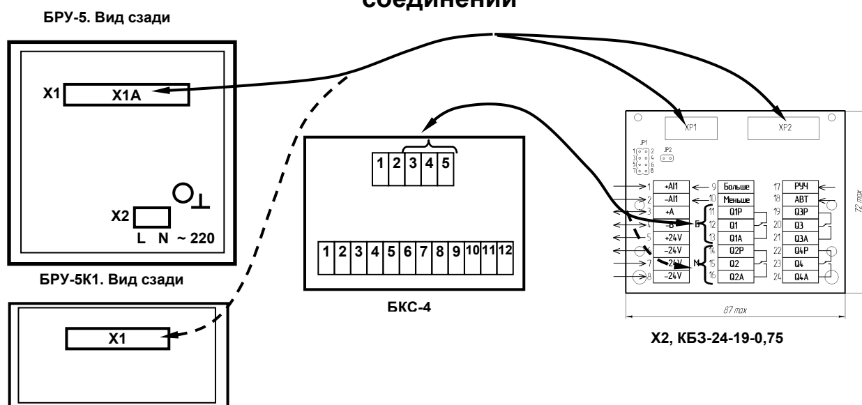
Рисунок Б.1 - Подключение клеммно-блочного соединителя КБ3-24-19-0,75 к блоку ручного управления БРУ-5 или БРУ-5K1
