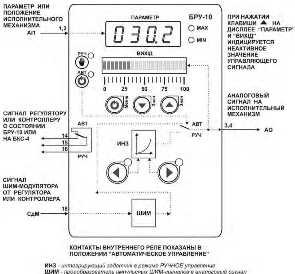
Рисунок 7.6.1 - Блок-схема режима 5
