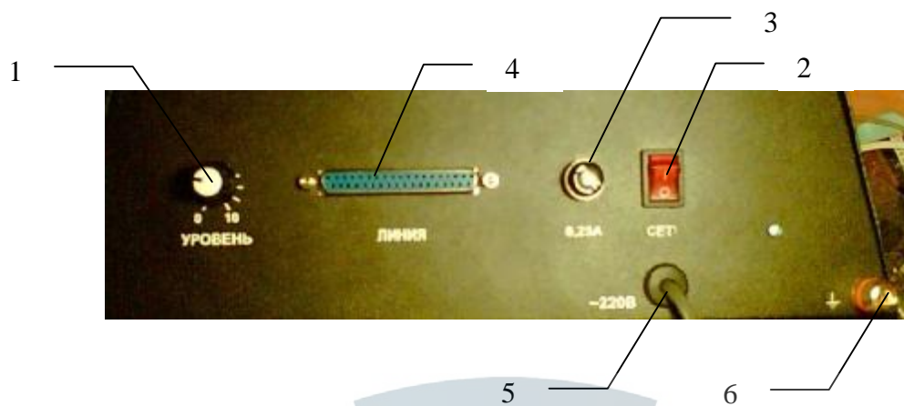
Рисунок 2 – Вид сзади
