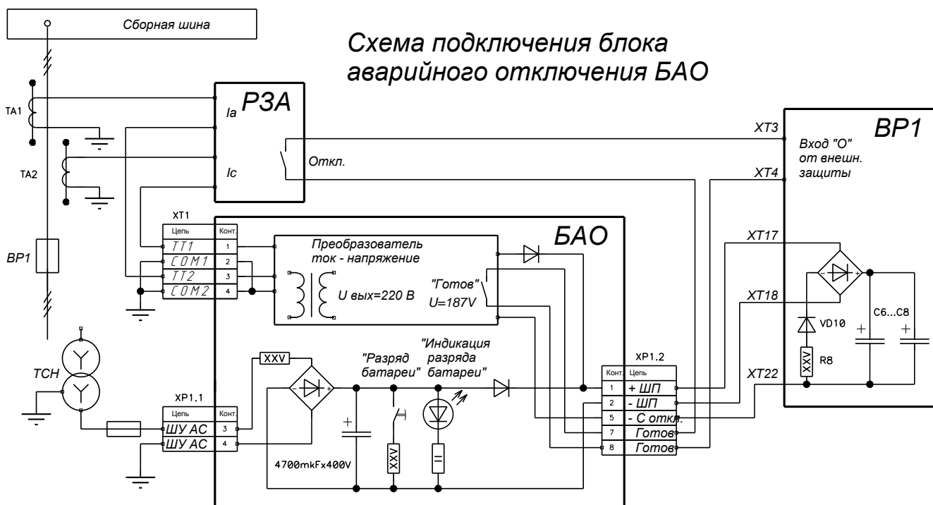
Рис.1. Схема подключения БАО
